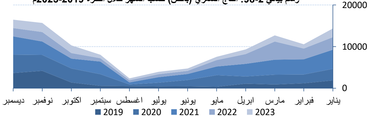
رسم بياني 2-98: انتاج الشعري (بالطن) حسب الشهر خلال الفترة 2019-2023م
